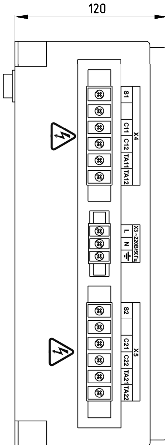
Рисунок А.1 – Внешний вид генератора. Боковая панель.
