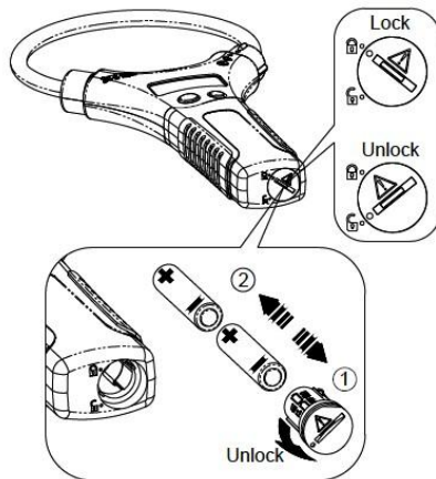
Рис. 7.1. Замена источников питания (на рис. указана модель серии sFlex D)
