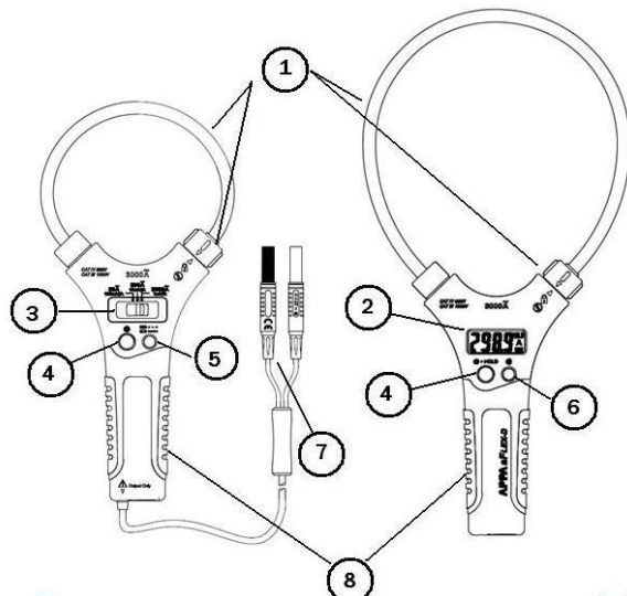
Рис. 5.1. Органы индикации и управления (слева - sFlex 10T, справа - sFlex 18D)
