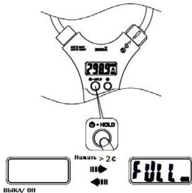
Рис.5.4 Включение питания и контроль заряда батарей
